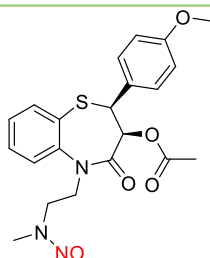
N-nitroso-N-desmethyl diltiazem
