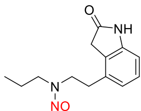
N-nitroso-despropyl-ropinirole
