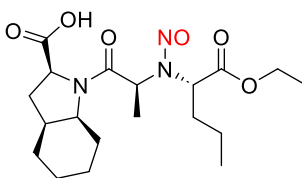
N-nitroso-perindopril
