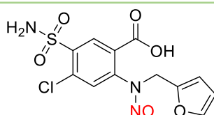
N-nitroso-furosemide
