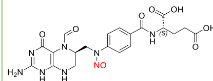
N-nitroso- levoleucovorin 2
