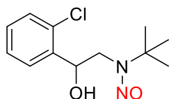
N-nitroso-tulobuterol
