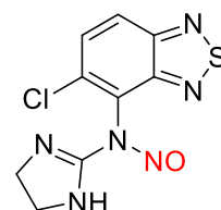
N-nitroso-tizanidine
