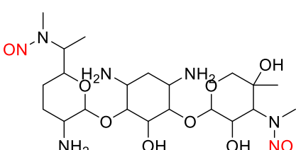
N-nitroso-gentamicin-2
