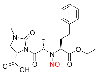
N-nitroso-lmidapril
