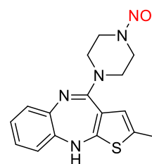
N-nitroso-N-desmethyl olanzapine
