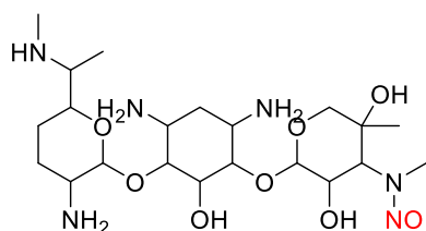
N-nitroso-gentamicin-1
