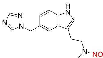
N-nitroso-desmethyl-Rizatriptan
