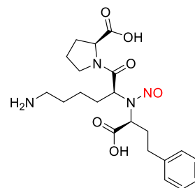
N-nitroso-lisinopril
