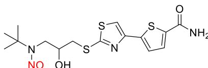
N-nitroso-arotinolol
