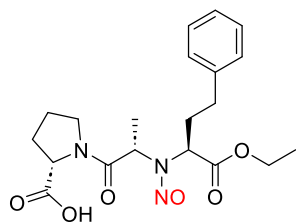
N-nitroso-enalapril
