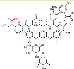
N-nitroso-vancomycin
