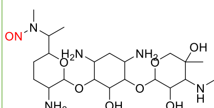
N-nitroso-gentamicin-3
