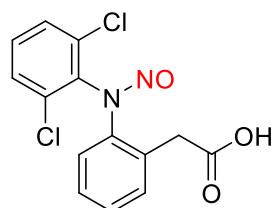
N-nitroso-diclofenac
