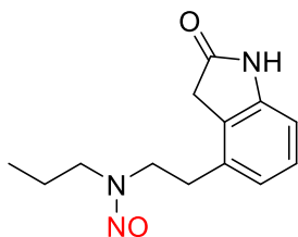
N-nitroso-despropyl-ropirole
