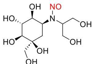
N-nitroso-voglibose
