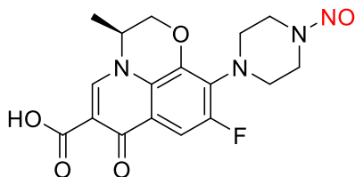
N-nitroso-levofloxacin
