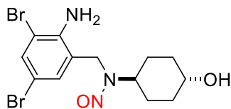
N-nitroso-ambroxol
