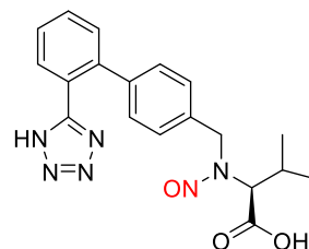
N-nitroso-desvaleryl- valsartan
