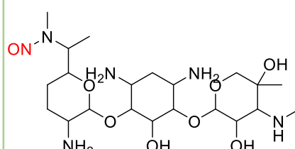
N-nitroso-gentamicin-3
