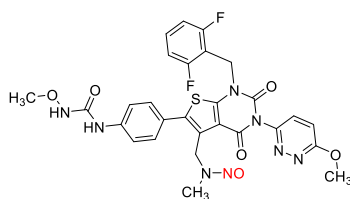
N-nitroso-desmethyl-relugolix
