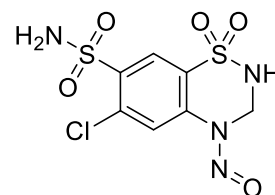
N-nitroso- hydrochlorothiazide
