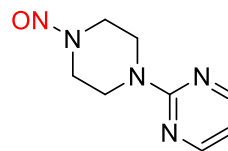
N-nitroso-buspirone Impurity 1
