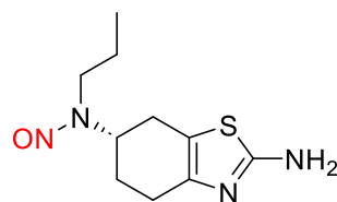
N-nitroso-pramipexole
