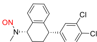
N-nitroso-sertraline
