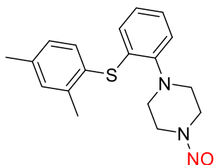
N-nitroso-vortioxetine
