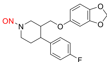
N-nitroso-paroxetine
