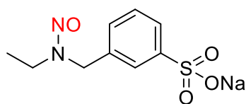
Sodium 3- ((ethyl(nitroso)amino)me thyl)benzenesulfonate
