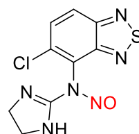
N-nitroso-tizanidine
