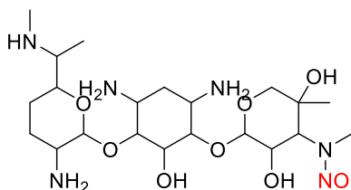
N-nitroso-gentamicin-1
